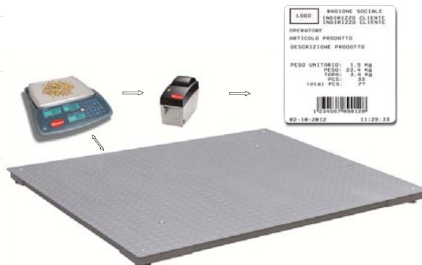
JCA bilancia remota collegabile a 2° piattaforma e a etichettatrice EZ2DT Jca Dual remote scale connection 2° floor platform and label printer EZ2DT
